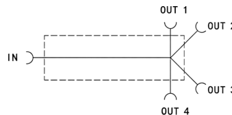
Lohkokaavio
